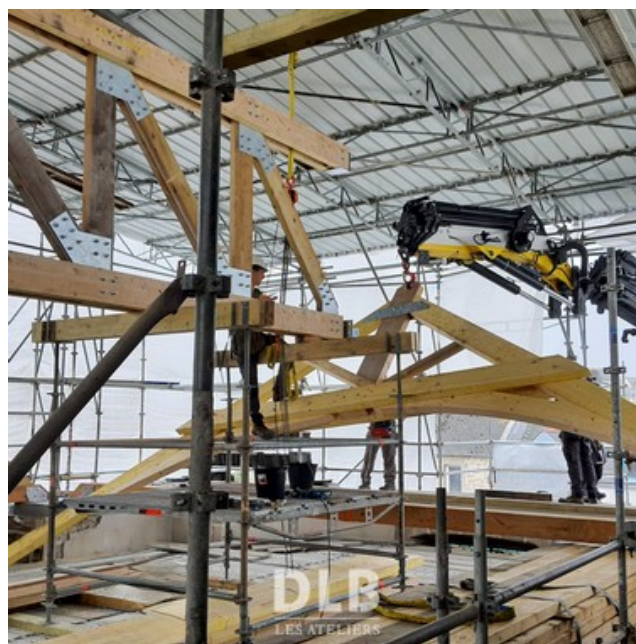
Assemblage de la ferme à la poutre maîtresse
